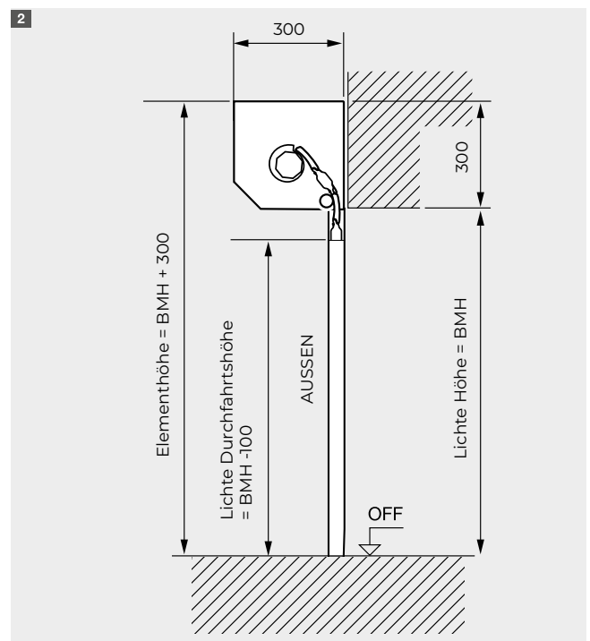
Einbau vor die Garagenöffnung, Außen-Rolltor
