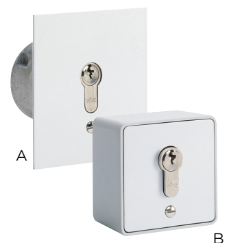
Schlüsseltaster ESU 40 / ESA 40 in Unterputz- (A) und Aufputz- ausführung (B), inklusive 3 Schlüsseln
